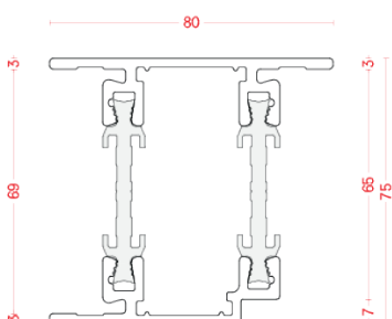
BT 7550L-08
