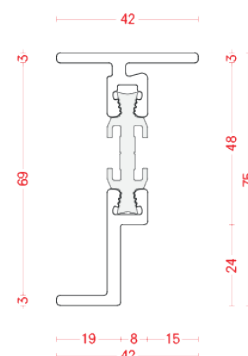
BT 7512HR-08
