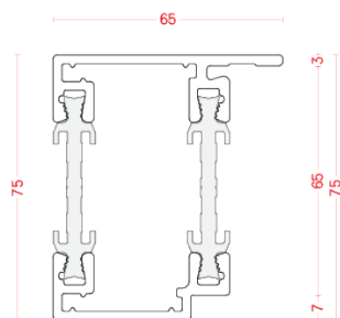
BT 7550L-08
