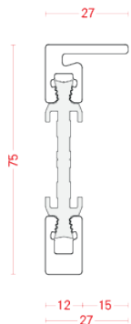
BT 7512L-08
