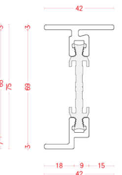
BT 7512HK-08
