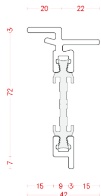
BT 8212TZ-08
