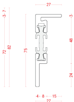
BT 7512LR-08
