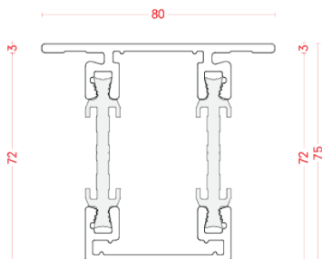
BT 7550TF-08
